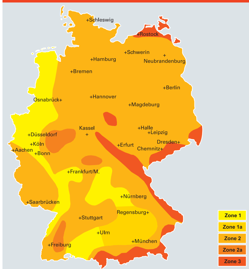
Abb. 1 Schneelasten
