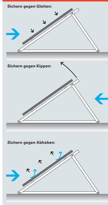
Abb. 6 Sichern der Sonnenkollektoren
