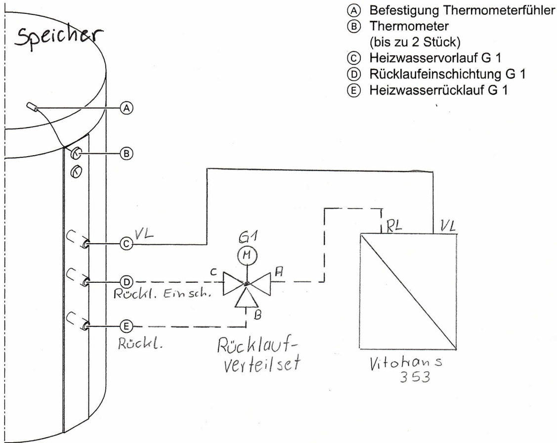
Abb. 1 Vorderseite, Ansicht ohne angebaute Solar-Divicon (Zubehör)
