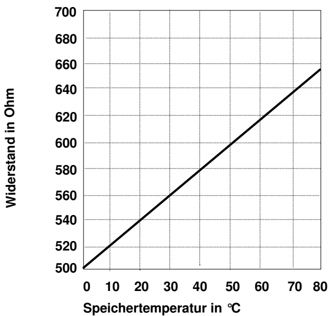
Speichersensur
