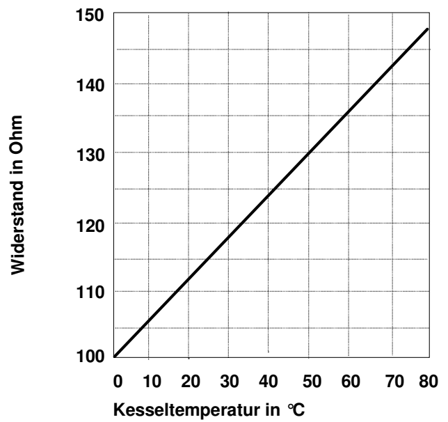
Kesseltemperatursensur, Vorlauftemperatursensur
